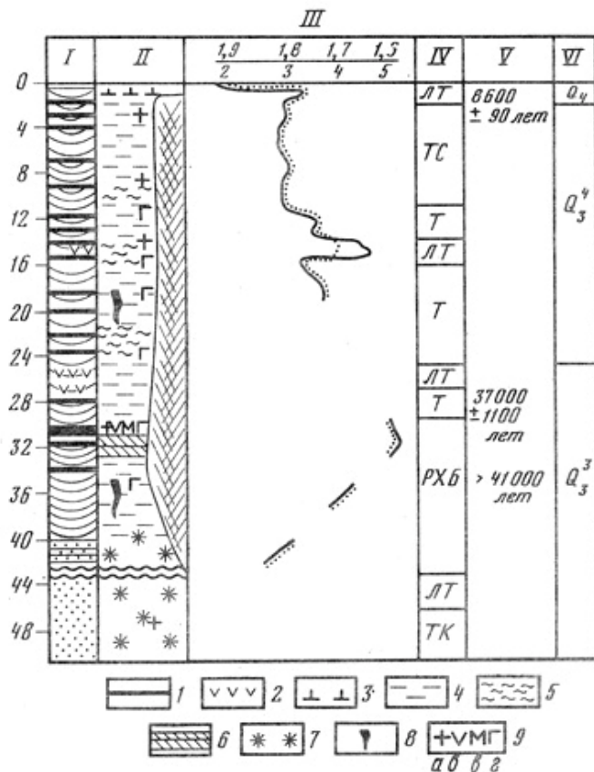
Рис. 3. Комплексная характеристика отложений Воронцовского Яра
