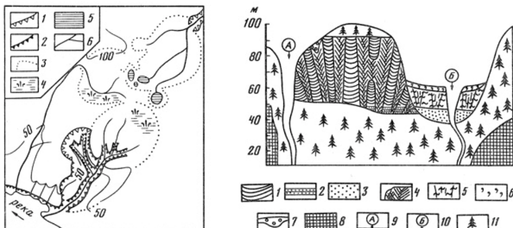
Рис. 1. Схема окрестностей Воронцовского Яра
