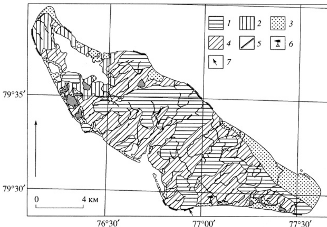
Рис. 2. Геоморфологическая схема острова Визе (Карское море)
