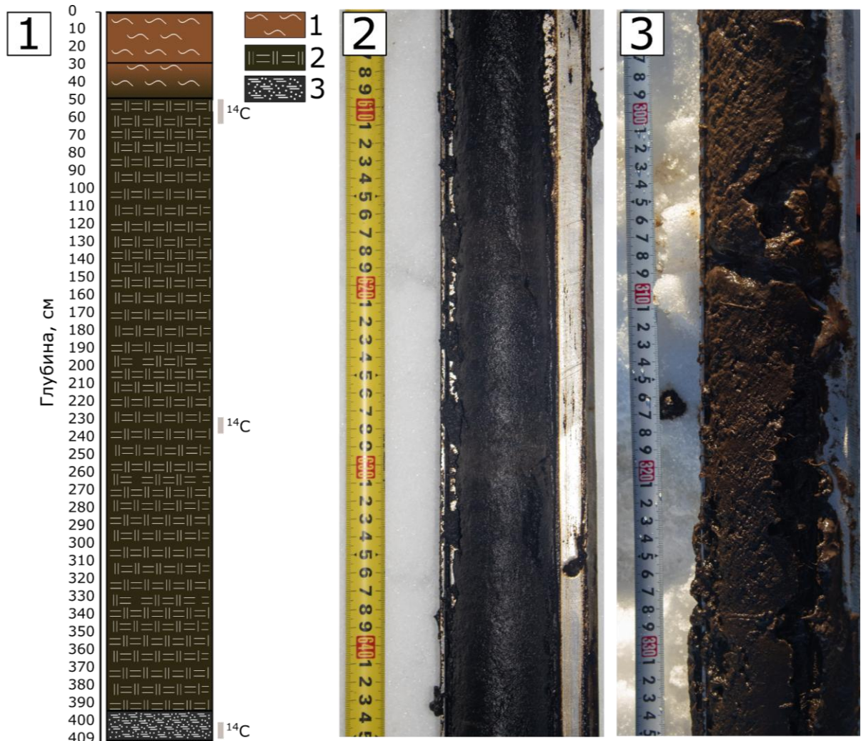
Рис. 2. 1. Литологическая колонка донных отложений оз. Змеиное: 1 - органомные илы, 2 - торфянистый сапропель, 3 - алевропелит; 2. Фрагмент керна №5 (3,09-4,09 м), нижняя часть торфянисто-сапропелевых отложений (3,30-3,74 м); 3. Фрагмент керна №1 (0,00-0,93 м), переходная зона (0,30-0,50 м) от торфянисто-сапропелевых к органомным илистым отложениям
