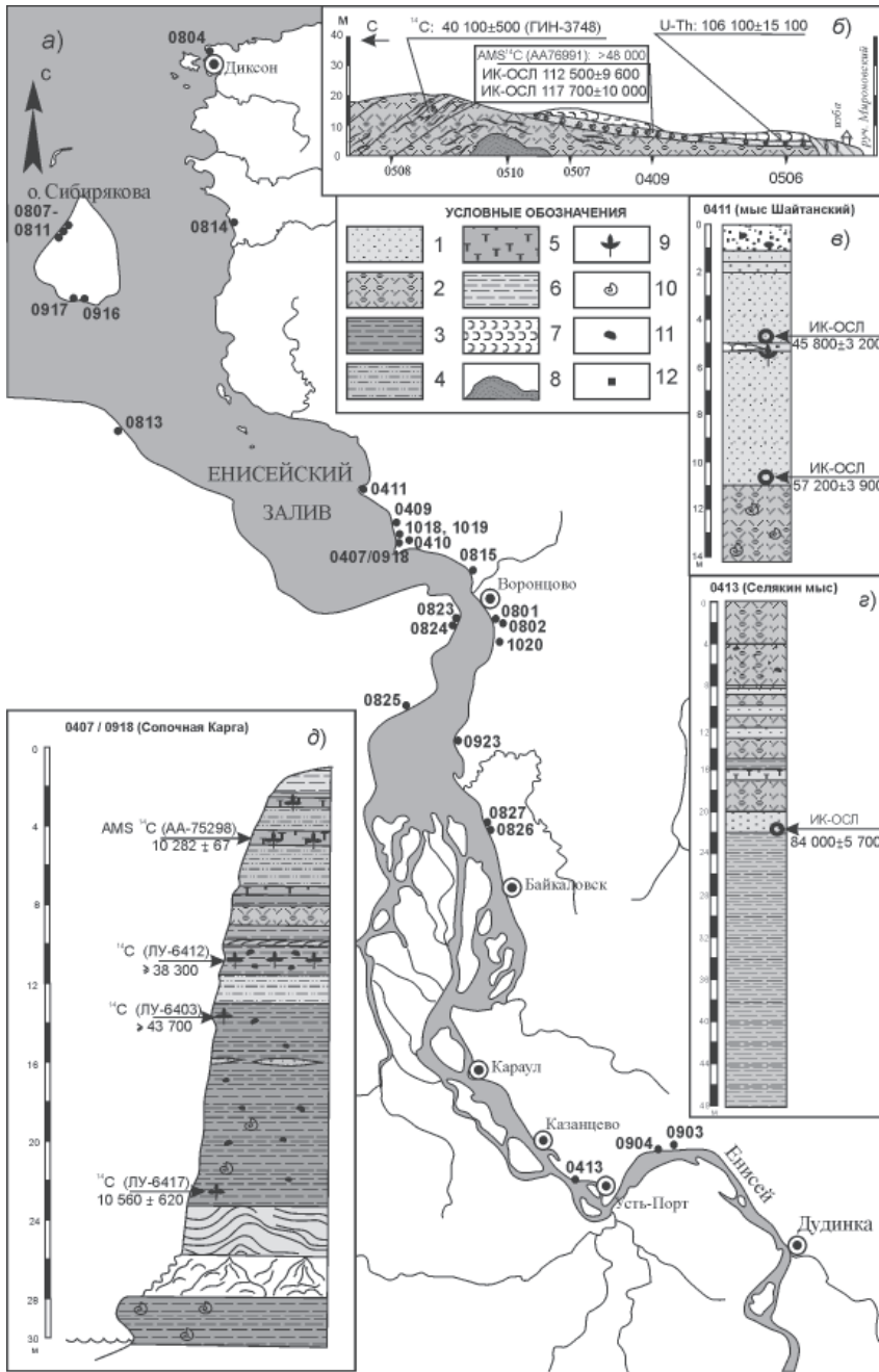
Рис. 1. Схема расположения датированных разрезов четвертичных отложений низовьев Енисея (а), геологический разрез восточного берега Енисейского залива у полярной станции Сопочная Карга (б), разрезы: мыса Шайтанский (в), мыса Селякина (з), Сопочная Карга (д)
