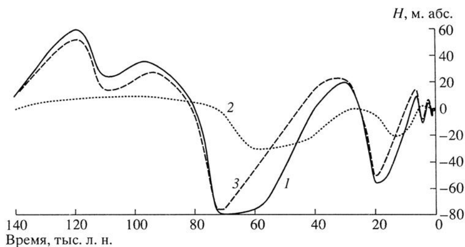
Рис. 2. Кривая колебания относительного уровня Восточно-Сибирского моря в последние 150 тыс. лет 1 – обобщающая кривая, 2 – гляциоэвстатическая составляющая, 3 – тектоническая составляющая
