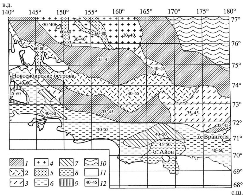
Рис. 1. Схема структурно-тектонического строения дна Восточно-Сибирского моря [по 1, упрощенная] с вероятными значениями внутриземного теплового потока [по 3]
