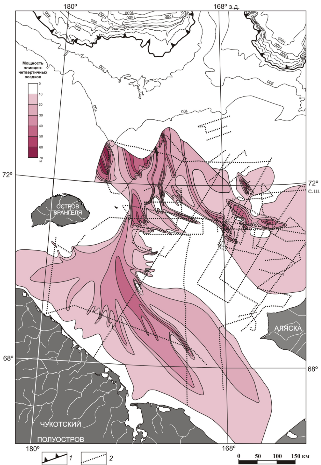
Рис. 4. Карта изобат верхнего сейсмокомплекса осадочного чехла Чукотского шельфа: 1 — бровка шельфа; 2 — использованные сейсмоакустические профили.
