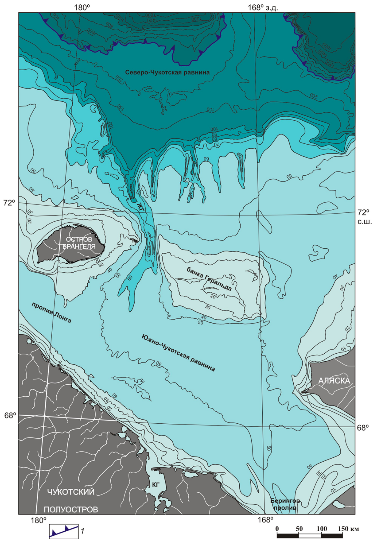
Рис. 1. Батиметрическая карта Чукотского шельфа: 1 — бровка шельфа; ЖГ — желоб Геральда; КГ — Колючинская губа.
