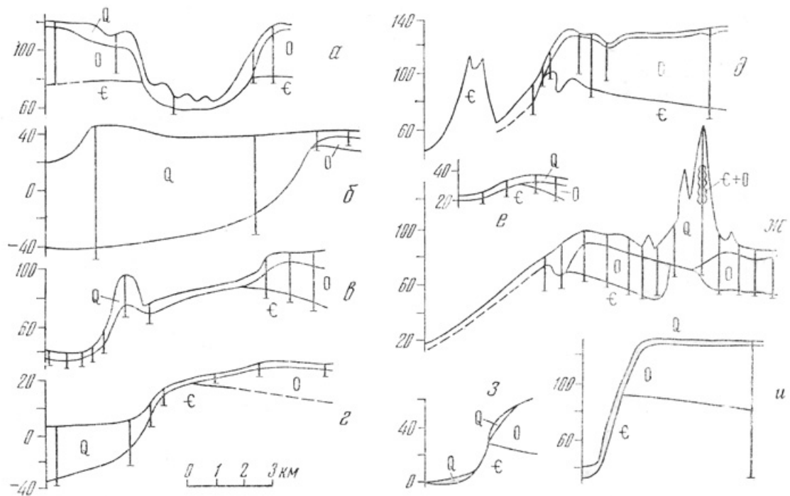
Рис. 1. Морфология и геологические разрезы района глинта Морфология глинта: а — Ропшинская ложбина, б — пос. Снявино и Михайловское, в — пос. Путилово, г — пос. Пулково, д — пос. Гостилицы, е — д. Захожье, ж — Дудергофские высоты, з — пос. Кунда, и — пос. Копорье
