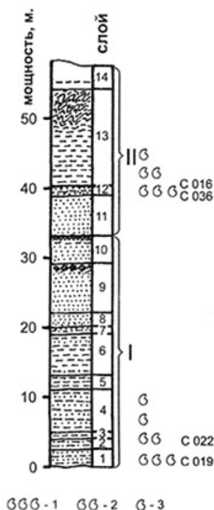
Рис. 4. Распространение раковин моллюсков в опорном разрезе мыса Каменного 1 – скопления раковин; 2 – уровни, где раковины встречаются часто; 3 – единичные находки раковин
