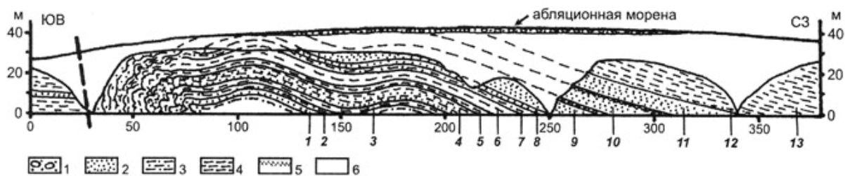
Рис. 3. Геологический профиль разреза морских и прибрежно-морских четвертичных отложений в т.н. А84 1 – галечники, 2 – пески, 3 – песчаные алевриты, 4 – алевриты, 5 – прослой торфа, 6 – нескрытые участки разреза. Под профилем обозначены номера слоев
